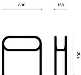
Accroche vélo
